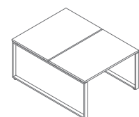
BOQ32 1200 / 1610 / 740 60 kg
